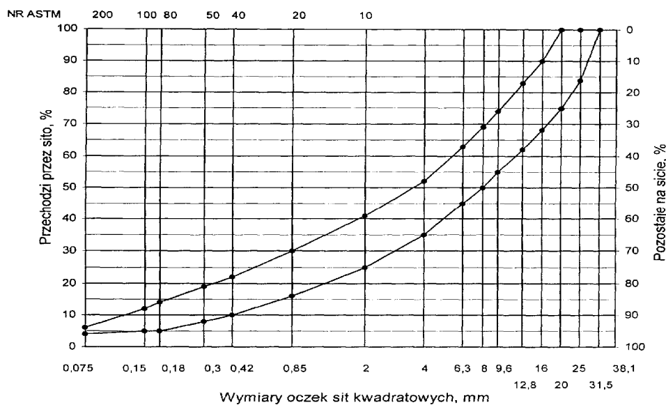
Rys. 12. Krzywe graniczne uziarnienia mieszanki mineralnej BA od 0 do 20 mm do warstwy wiążącej, wyrównawczej i wzmacniającej nawierzchni drogi o obciążeniu ruchem KR3
