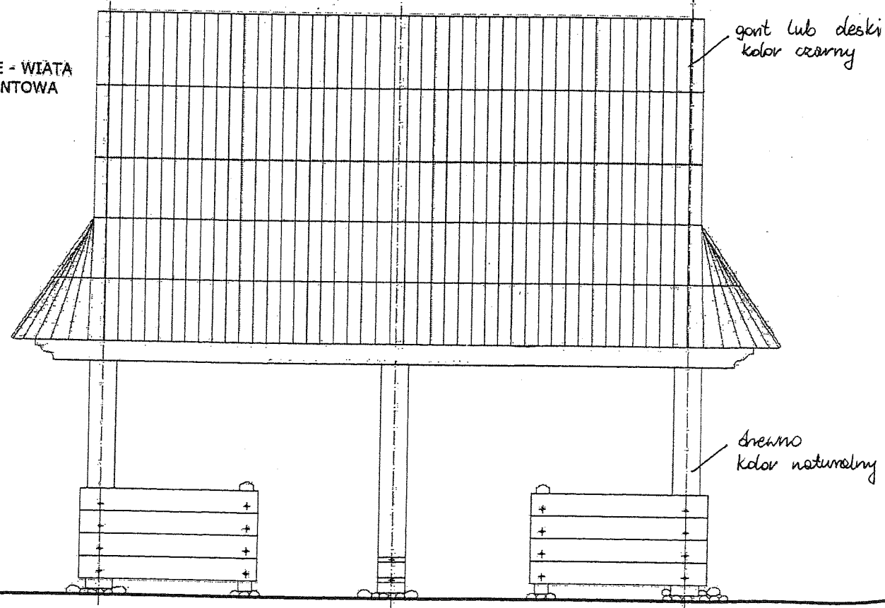
1. ZADASZENIE - WIATA ELEWACJA BOCZNA
